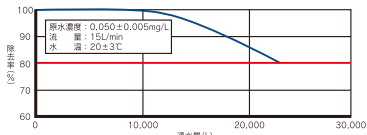
CAT(シマジン)ろ過能力試験
