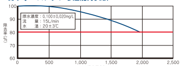
2-MIB(カビ臭)ろ過能力試験
