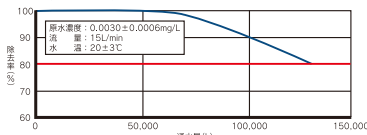
総トリハロメタンろ過能力試験
