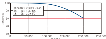
溶解性鉛ろ過能力試験
